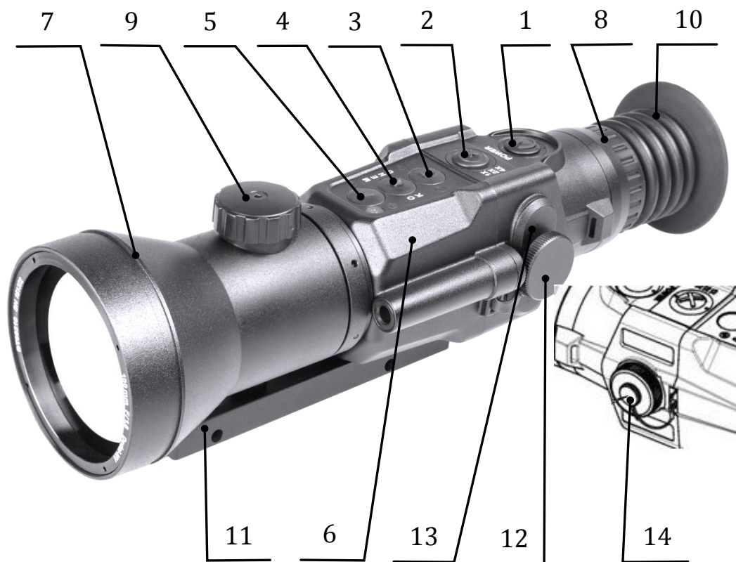
Рисунок 1 – Внешний вид прицела и органы управления
